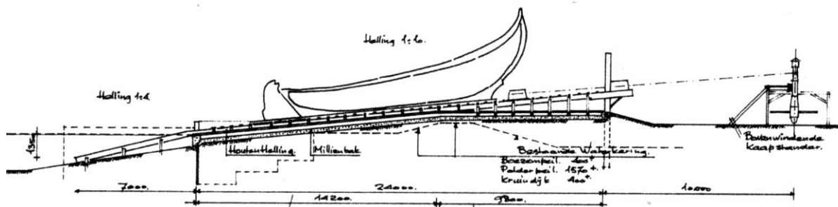
Scheepshelling geschikt voor het 'hellingen' van historische schepen...
