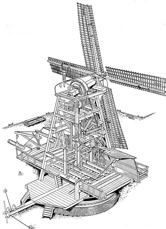
Perspectieftekening van de paltrok zaagmolen.
