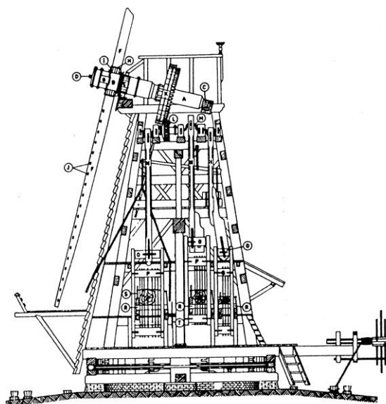
Doorsnede van de 'Zaanse' paltrok.
